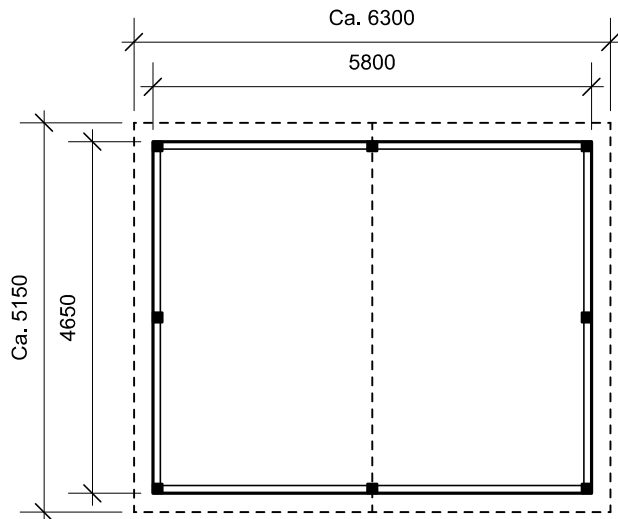
Plantegning
