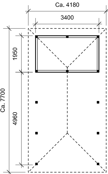
Plantegning
