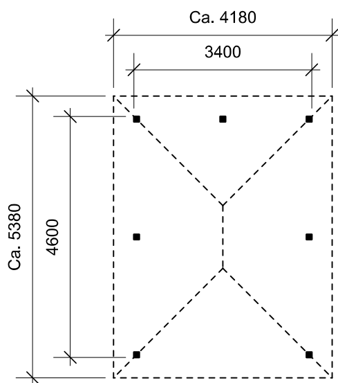
Plantegning
