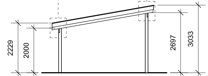
Gavl
