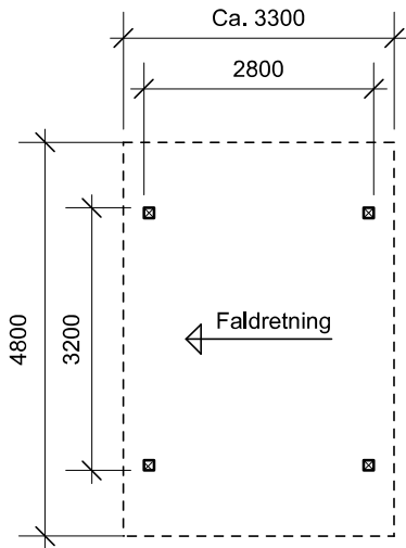
Plantegning
