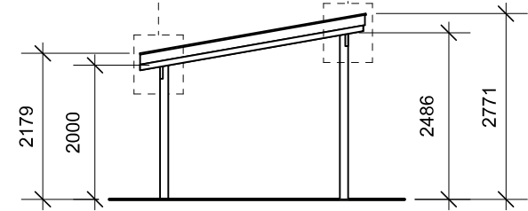
Gavl
