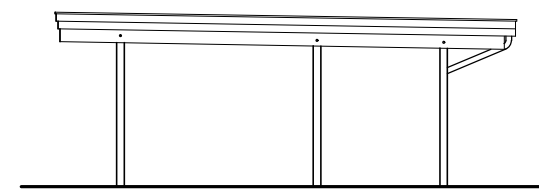
Facade - højre
